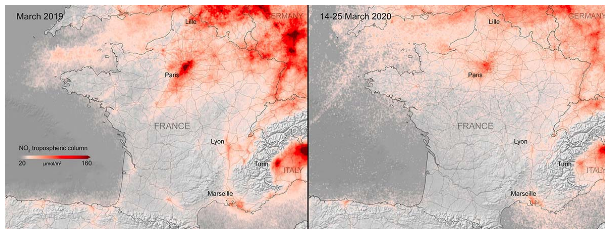
Figure 3. Comparaison des concentrations atmosphériques en NO 2 au-dessus de la France entre mars 2019 (sans confinement) et mars 2020 (période de confinement). Les données proviennent des observations du satellite Sentinel-5P du programme Copernicus (source : https://copernicus.cnes.fr/fr/covid-19-chute-de-la-pollution-en-europe-avec-le-confinement )
