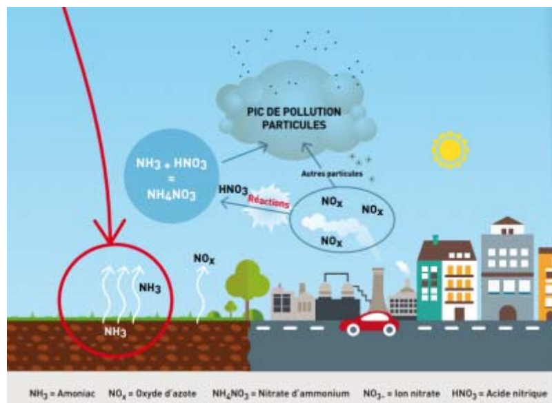
Figure 6. Cycles de réactions chimiques dont l'ammoniac \text{NH}_3 est le précurseur. En présence de \text{NO}_x à proximité, il est peut être responsable de pics de pollution aux particules fines. Source : https://www.atmo-auvergnerhonealpes.fr/article/agriculture-et-qualite-de-lair
