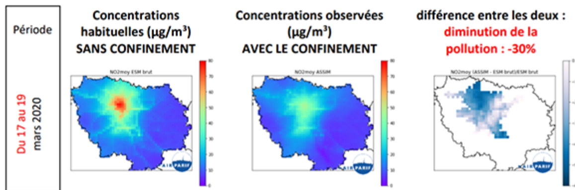
Figure 4 : Evolution de la concentration en dioxyde d'azote dans la région Ile de France entre une moyenne dans une situation sans confinement et la moyenne des trois premiers jours de confinement du 17 au 19 mars 2020 (source : AirParif).
