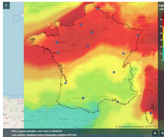
Figure 5. Pic de pollution aux particules fines observé dans le nord de la France le samedi 28 mars 2020. Données Prev'air
