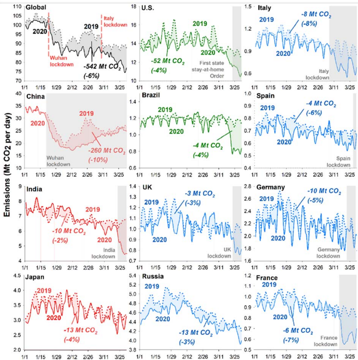
Figure 1. Evolution des émissions de CO 2 , en millions de tonnes par jour, en 2019 et en 2020. La partie grisée correspond à la période de confinement.
