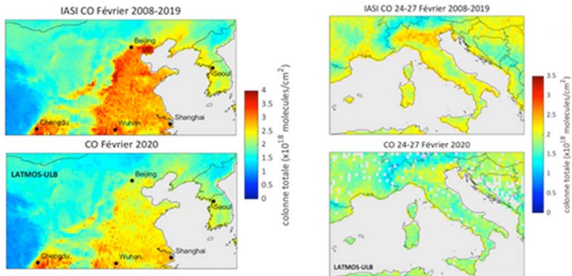
Figure 2 : Comparaison des concentrations atmosphériques en CO au-dessus de la Chine et de l'Italie entre la moyenne 2008-2019 (sans confinement) et février 2020 (période de confinement). Les données proviennent des observations de la sonde IASI.
